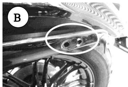
両面テープ②を貼付ける。
