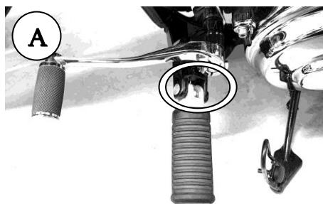
ピン/E クリップを取外します。
