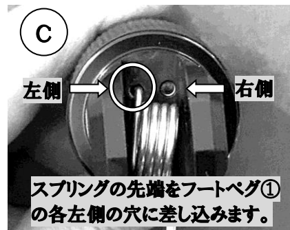
スプリングの先端をフートペグ①に差し込みます。
