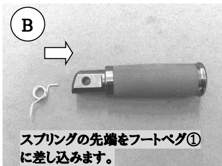
スプリングの先端をフートペグ①の各左側の穴に差し込みます。
